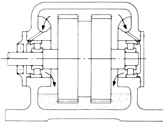
그림 12.6 비산급유법의 예
