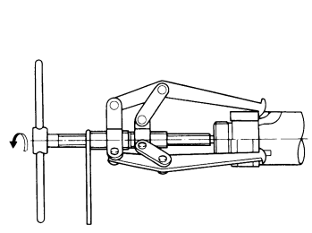
그림 14.13 인발치구에 의한 내륜의 해체(2)
