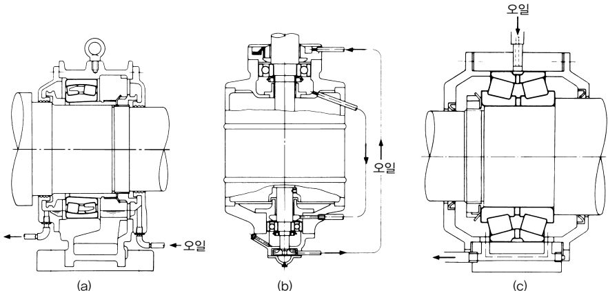
그림 12.7 순환급유법의 예
