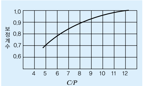
그림 6.1 베어링하중의 크기에 따른 허용회전수의 보정
