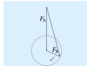
그림 5.8 회전하중과 정지하중
