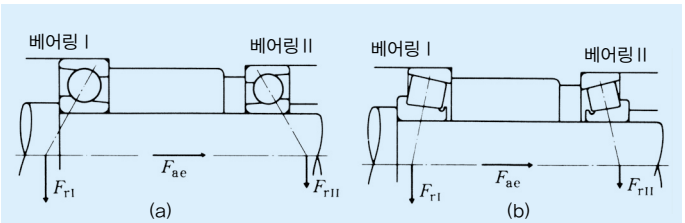
그림 5.12 각 베어링에 걸리는 하중의 관계
