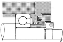
(a) 액셀라비린스
