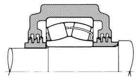
(c) 조심축의 라비린스
