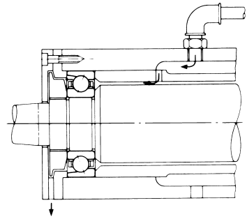
그림 12.9 분무급유법의 예
