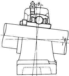
그림 3.5 볼 베어링유니트의 허용조심각
