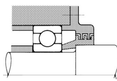
(b) 레이디얼라비린스
