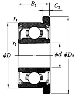
시일드형 ZZ · ZSS
