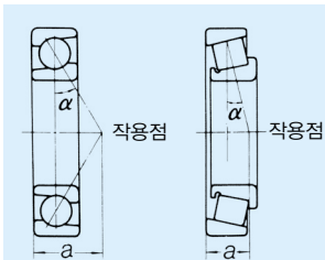
그림 5.11 하중의 작용점
